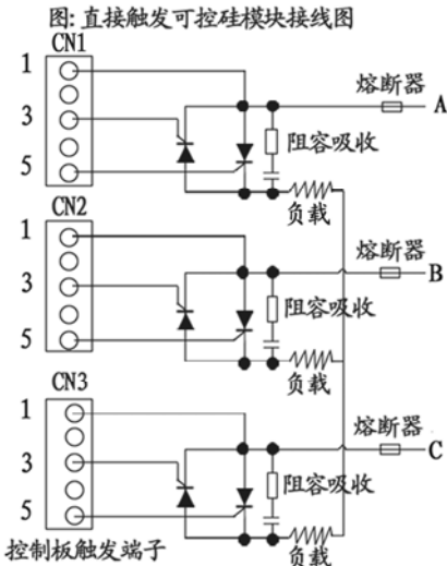
图 2-2 控制板与可控硅接线方式
