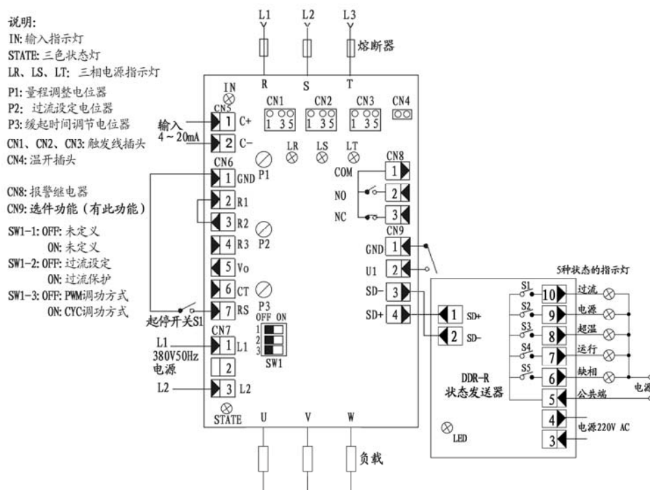
图 2-1-3 星型中心不接地负载自动方式接线图、控制板端子位置图、选件 DDR-R 接线图
