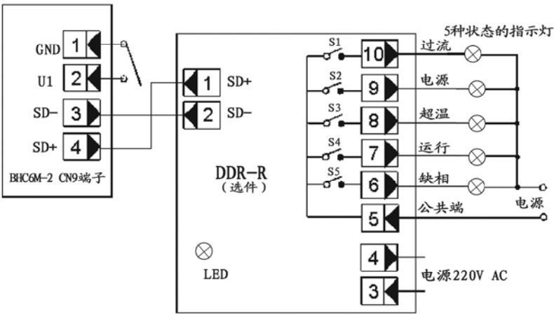
图 2-3 DDR-R 接线图
