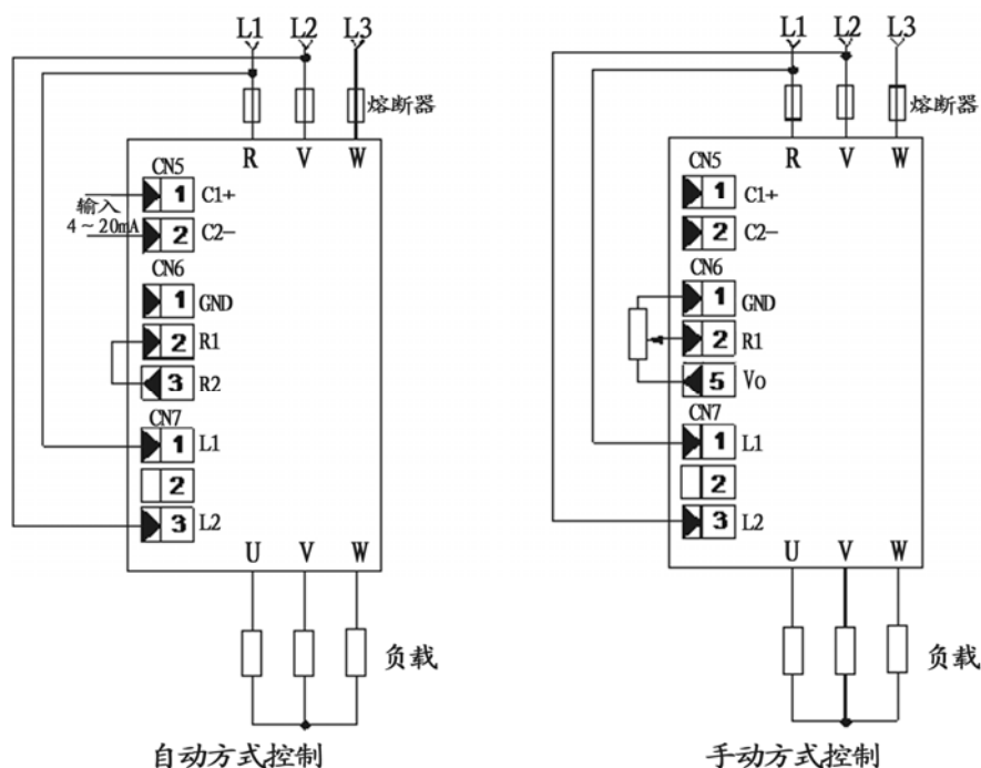
图 2-4 手动及自动时接线方式
