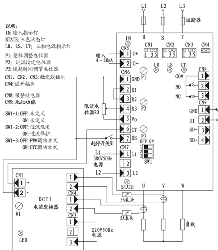
图 2-1-2 自动控制带限流、过流保护功能
