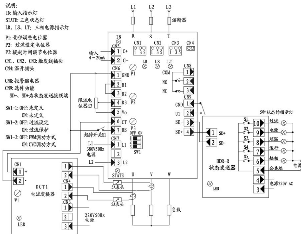
图 2-1-4 星型中心不接地负载自动方式接线图、控制板端子位置图、选件 DCT1、选件 DDR-R 接线图
